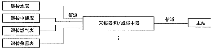
图 A.1 抄表系统准确度试验原理线路图
